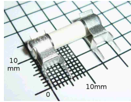
Fuseholder5x20_horiz_open_Inline_Type - L_RevC_Date24Feb2011
