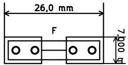
Fuseholder5x20_horiz_open_Inline_Type - L_RevC_Date24Feb2011
