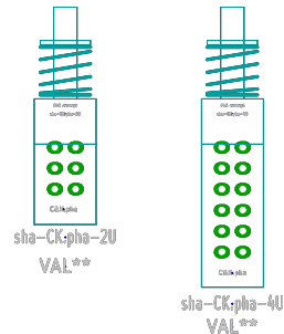
C&K PHA series matrice 2,5mm x écartement 2,5mm
