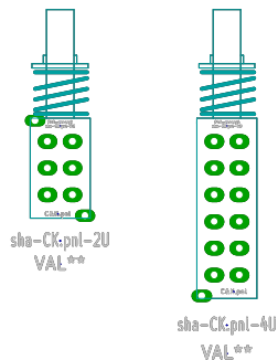
C&K PNL series metal matrice 3,2mm x écartement 3mm
