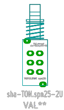
TONELUCK SPN25 series metal matrice 2,5mm x écartement 2,5mm
