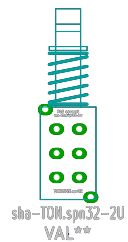
TONELUCK SPN32 series metal matrice 3,2mm x écartement 3mm
